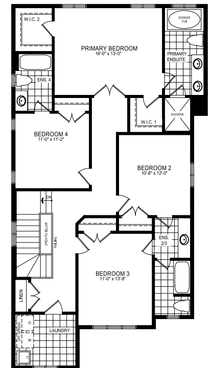
ELEV. A
